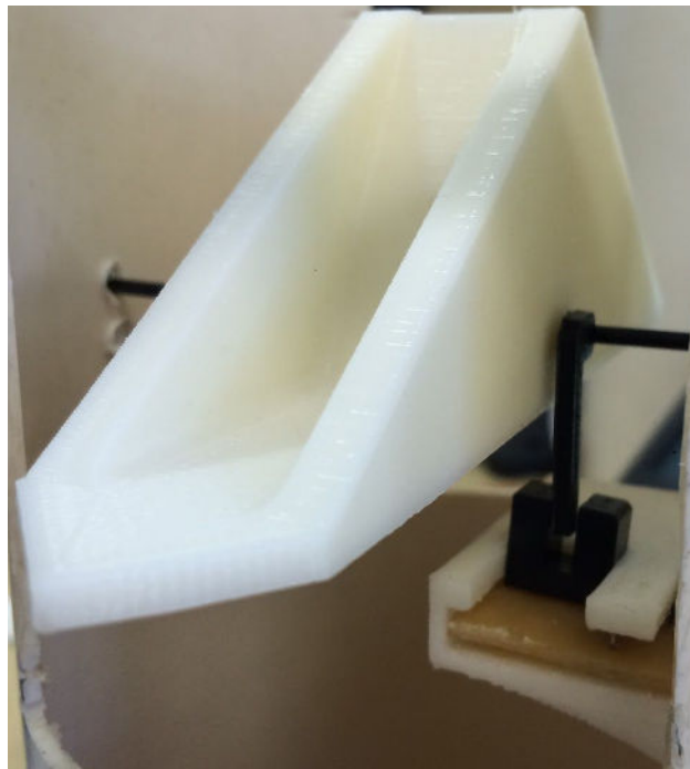
Figura 3: Balança, chave de interrupção e circuito do primeiro modelo do pluviômetro. Fonte: Elaboração própria
